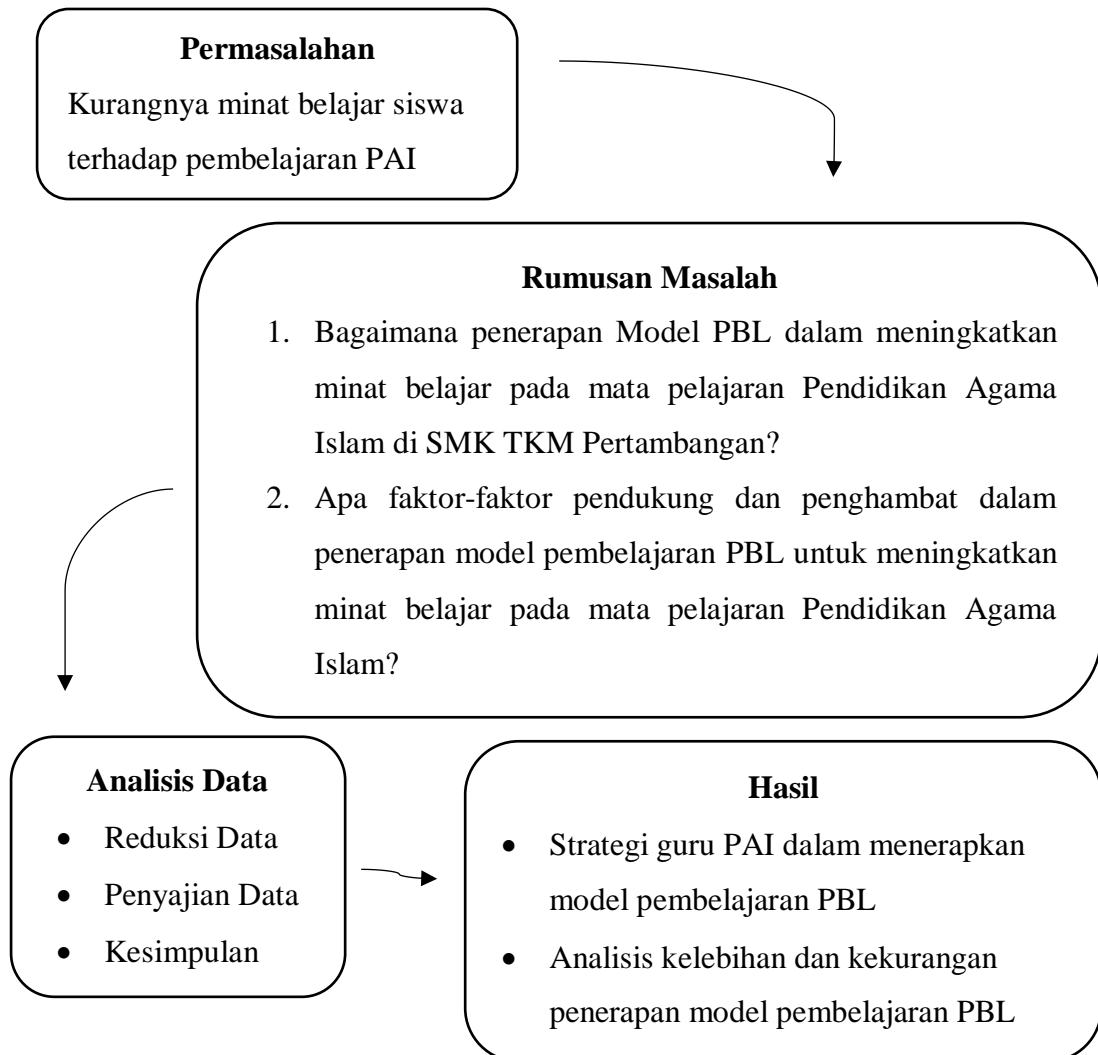
Gambar 3.1 Kerangka Pemikiran
