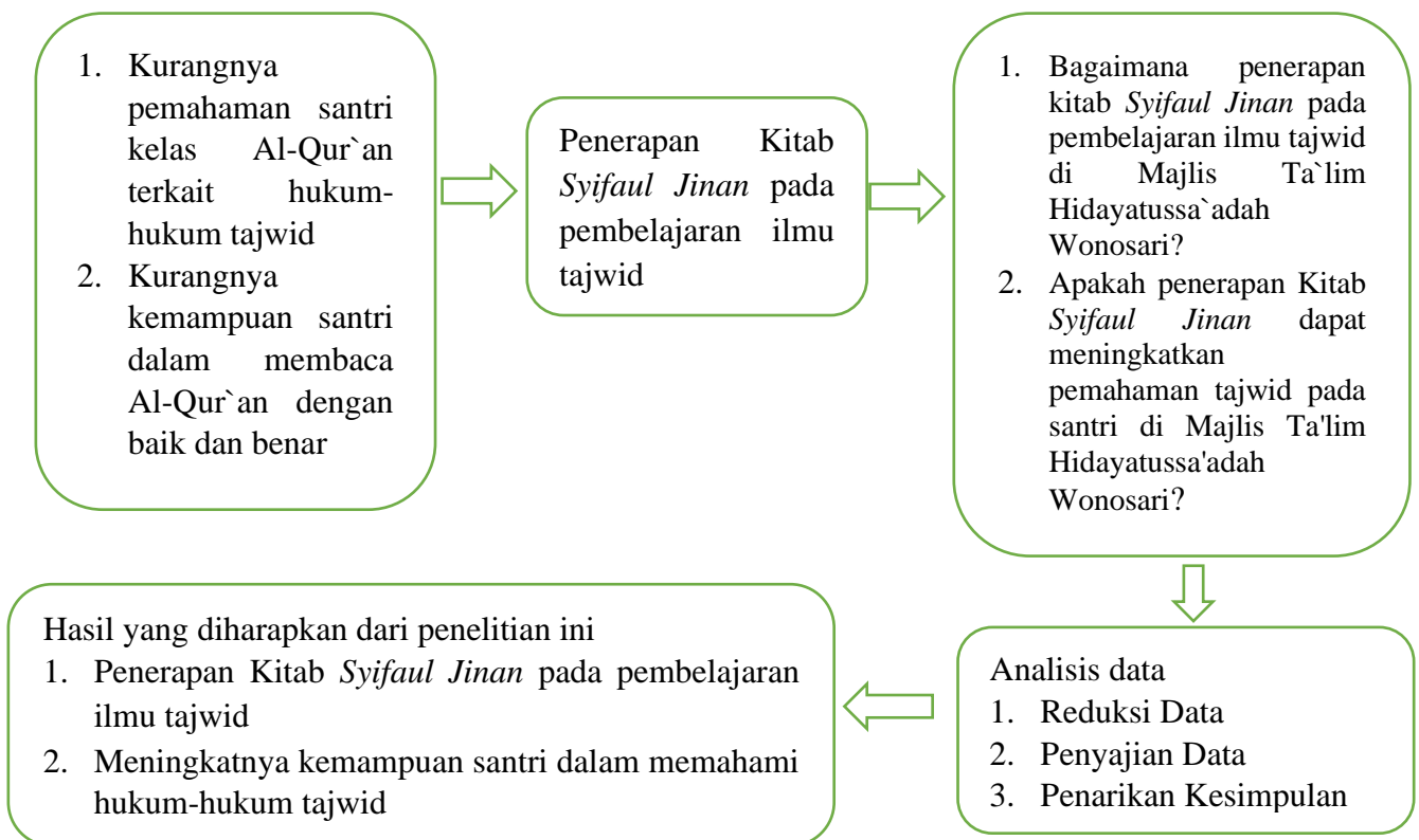
Gambar 3.1 Kerangka Pemikiran
