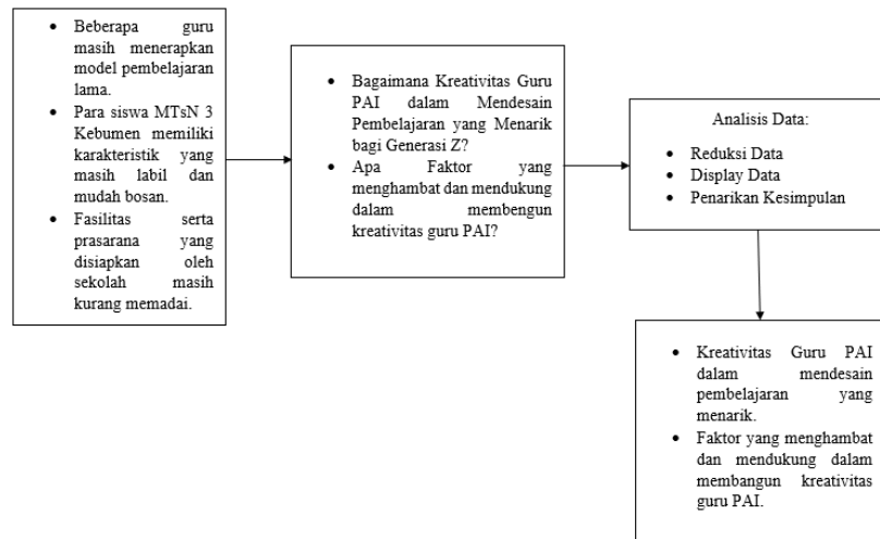
Gambar 3. 3 Kerangka Pemikiran
